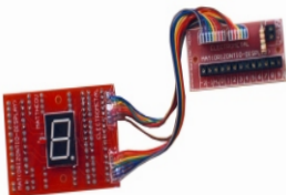
ΠΛΑΚΕΤΑ DISPLAY ΟΡΙΖΟΝΤΙΟ ΚΩΔΙΚΟΣ: 3304
